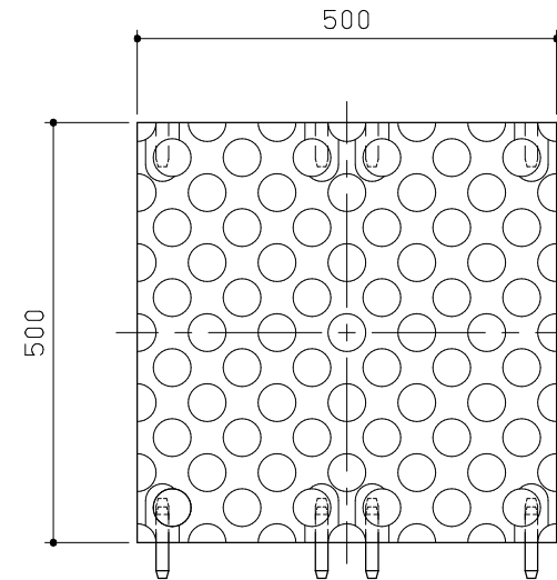
下面図 S = 1 / 10
