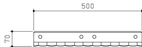
正面図 S = 1 / 10
