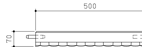
側面図 S = 1 / 10
