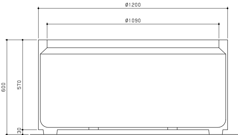
断面図 S = 1 / 10
