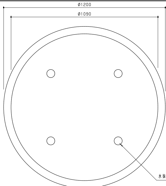
平面図 S = 1 / 10
