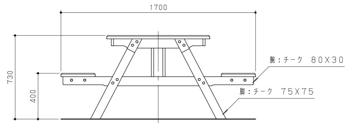
側面図 S=1/20
