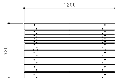
平面図 S = 1 / 20
