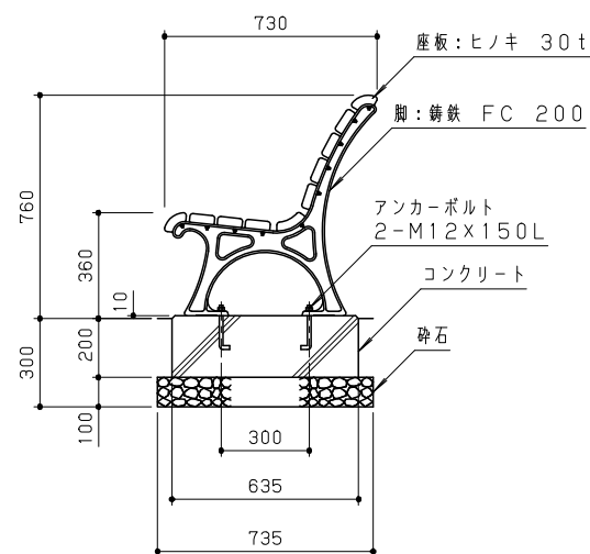
側面図 S = 1 / 20
