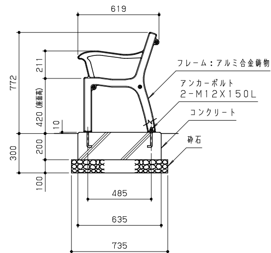
側面図 S=1/20
