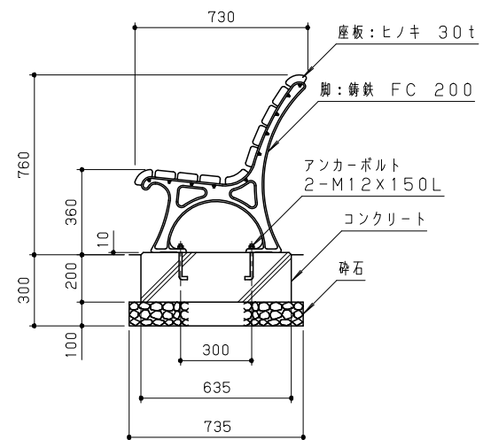
側面図 S = 1 / 20
