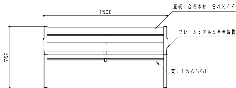
立面図 S=1/20
