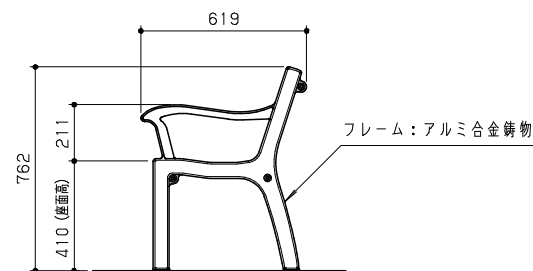
側面図 S=1/20
