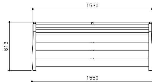
平面図 S=1/20
