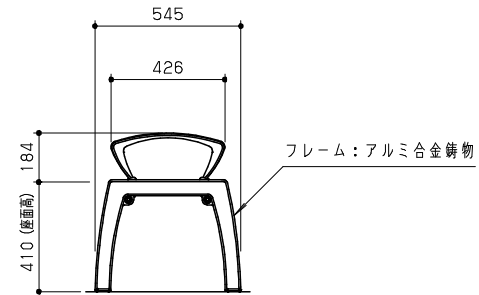
側面図 S = 1 / 20
