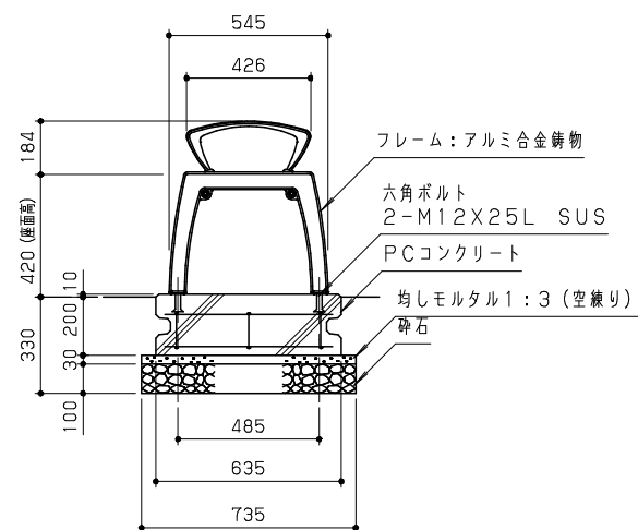
側面図 S=1/20
