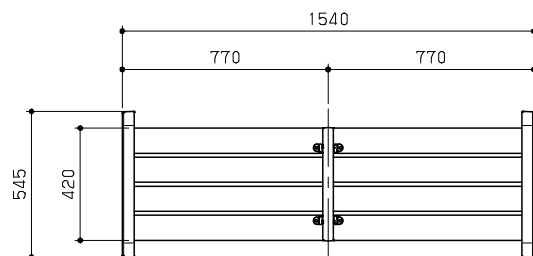
平面図 S=1/20
