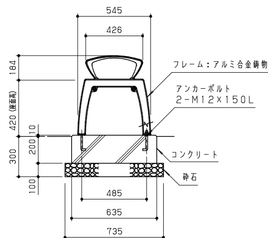
側面図 S = 1 / 20
