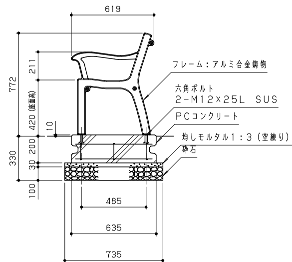
側面図 S = 1 / 20
