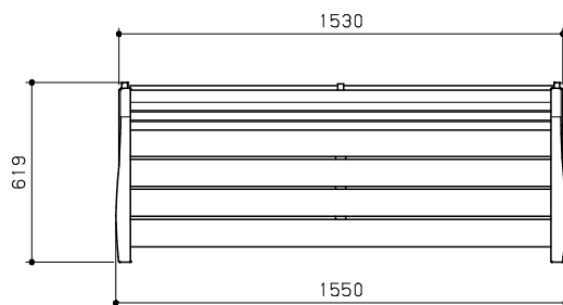
平面図 S = 1 / 20
