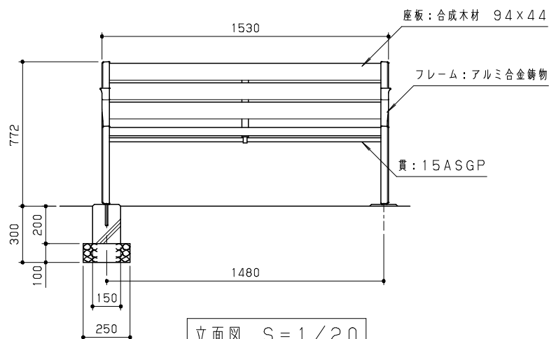
立面図 S = 1 / 20
