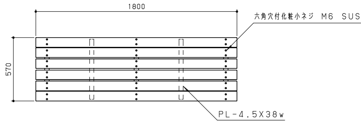
平面図 S=1/20
