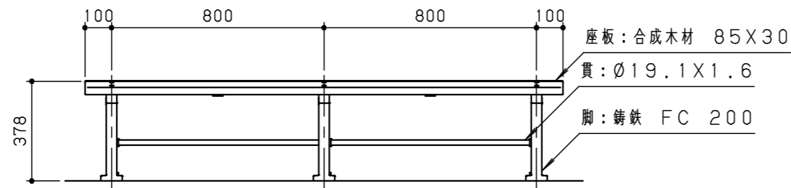
正面図 S=1/20
