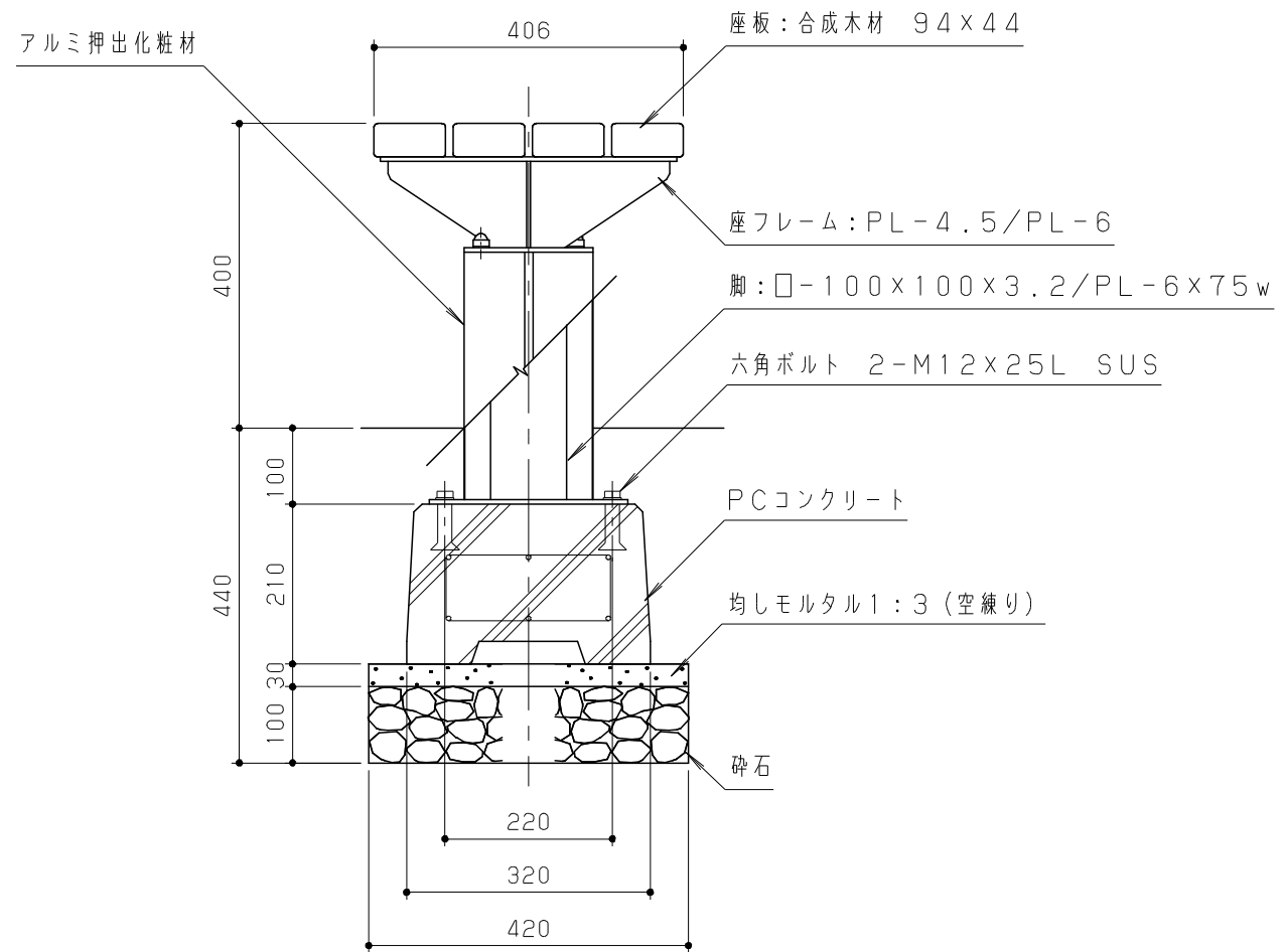
側面図 S = 1 / 10
