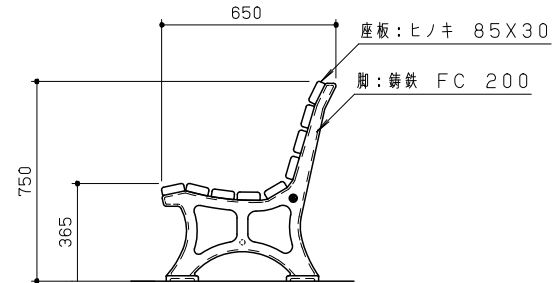
側面図 S = 1 / 20
