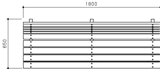
平面図 S = 1 / 20
