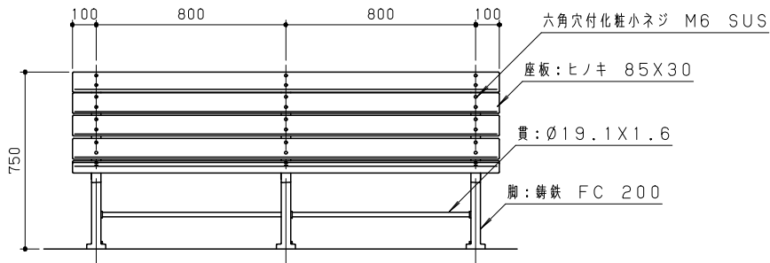
正面図 S = 1 / 20
