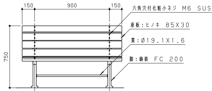
正面図 S = 1/20
