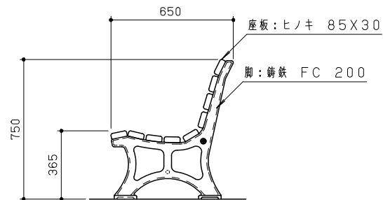
側面図 S = 1/20
