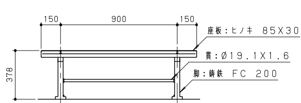
正面図 S = 1/20
