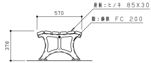
側面図 S = 1/20
