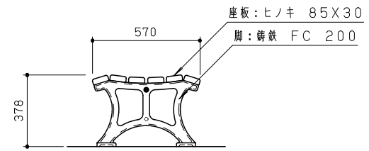
側面図 S=1/20
