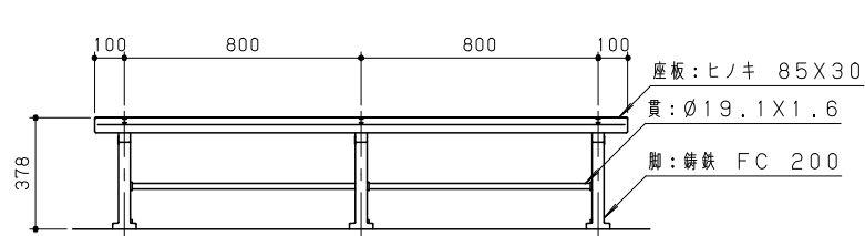
正面図 S=1/20
