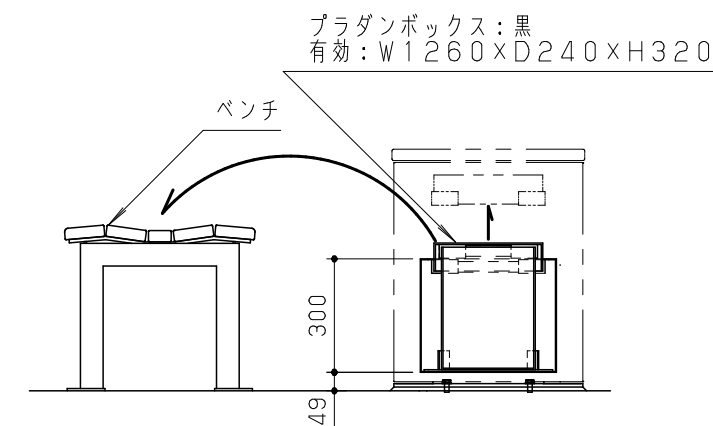
収納ボックス断面図 S = 1 / 20
