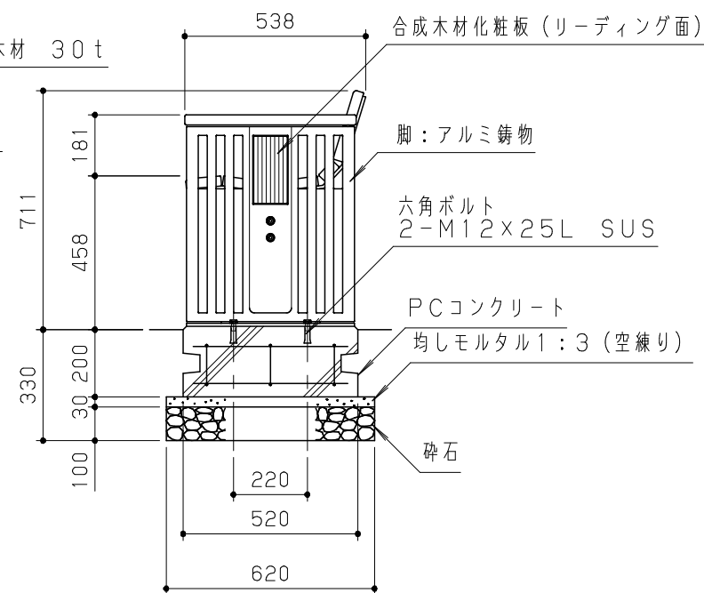
側面図 S = 1 / 20
