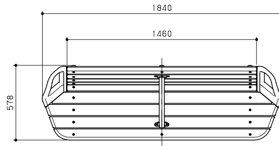
平面図 S = 1 / 20
