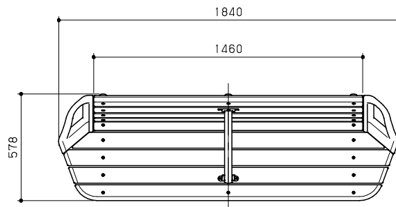
平面図 S=1/20
