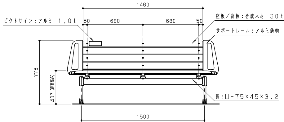
立面図 S = 1 / 20
