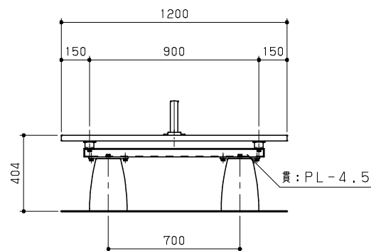
立面図 S = 1 / 20
