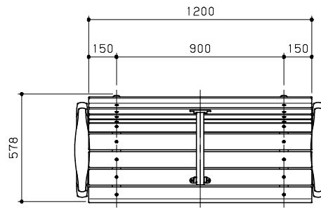
平面図 S=1/20
