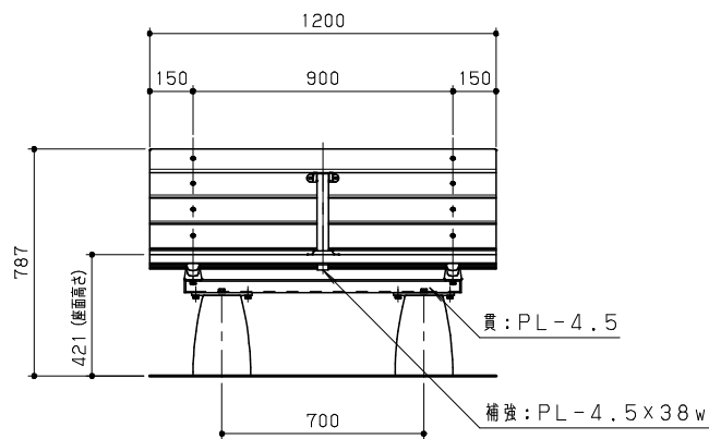
立面図 S = 1 / 20
