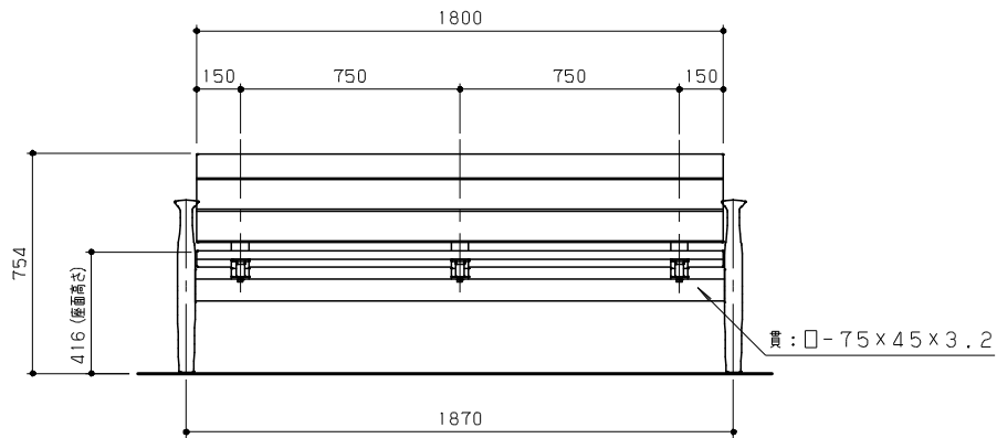
立面図 S = 1/20
