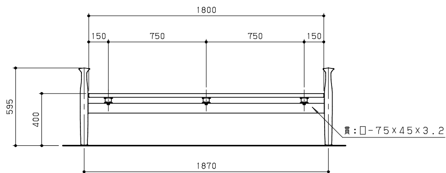
立面図 S = 1 / 20
