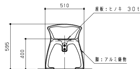
側断面図 S = 1 / 20
