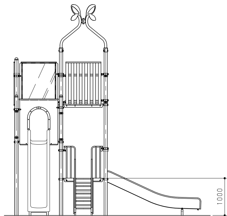
D 視立面図 S = 1 / 6 0
