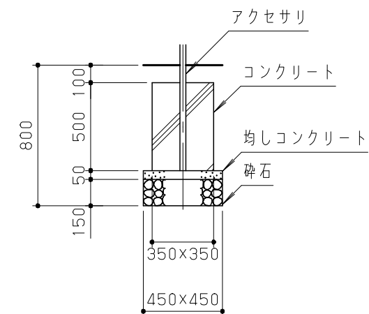
基礎標準断面詳細図 S = 1 / 30
