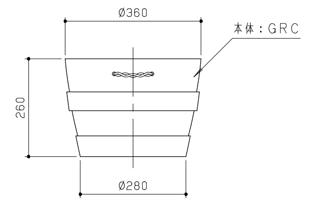
側面図 S = 1 / 10
