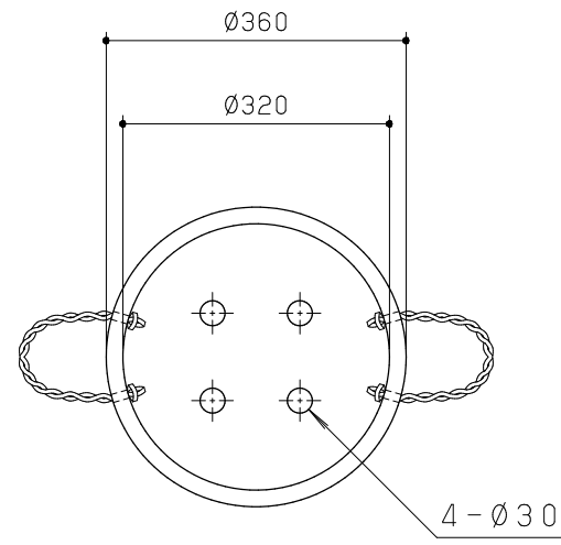
平面図 S = 1 / 10
