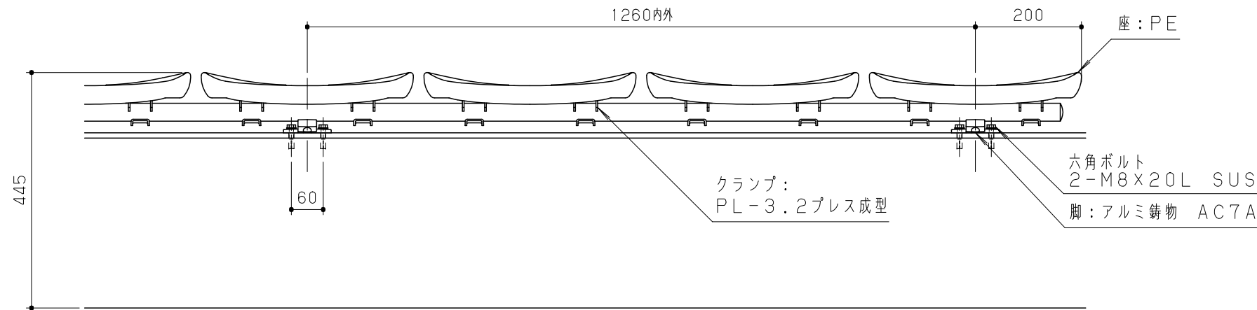
正面図 S = 1 / 10
