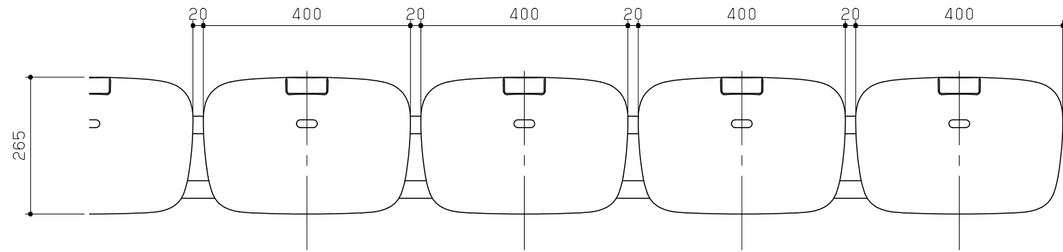
平面図 S = 1 / 10
