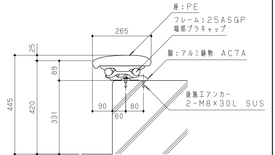
側面図 S = 1 / 10
