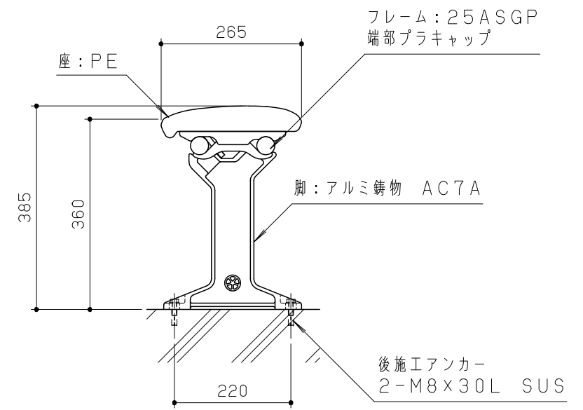
側面図 S = 1 / 10
