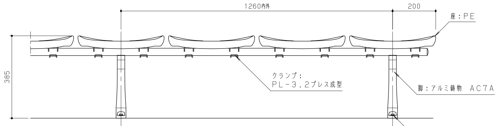
正面図 S = 1 / 10
