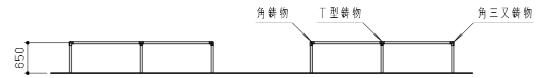
側面図 S = 1/80
