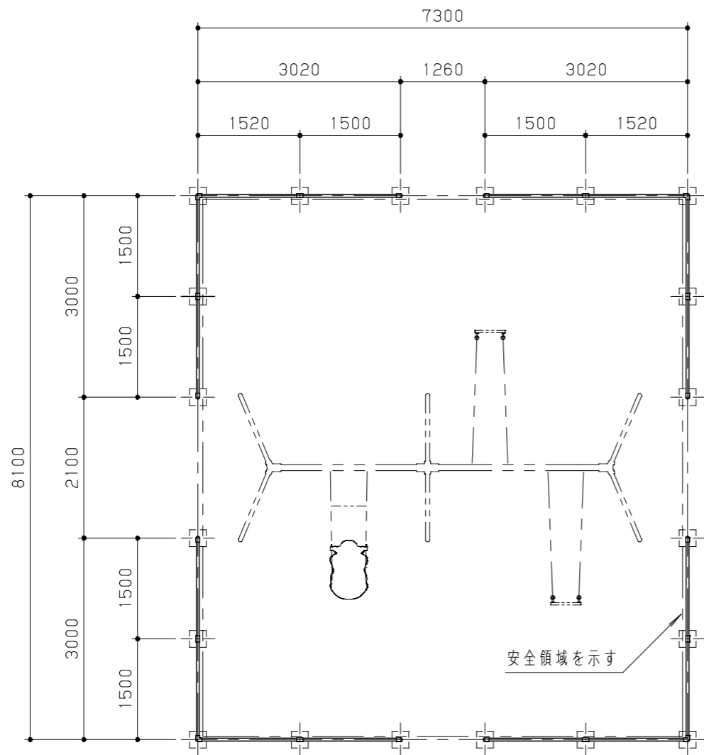
平面図 S = 1/80
