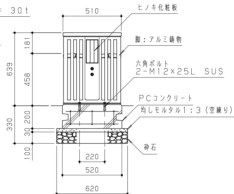
側面図 S = 1 / 20
