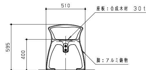
側断面図 S = 1 / 20
