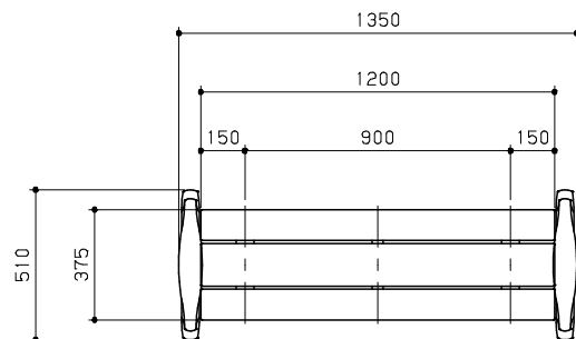
平面図 S = 1 / 20
