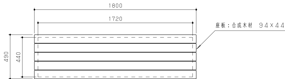
平面図 S = 1 / 20
