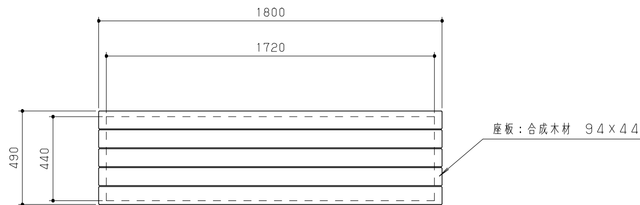
平面図 S = 1 / 20
