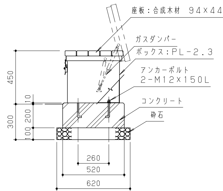
側面図 S = 1 / 20
