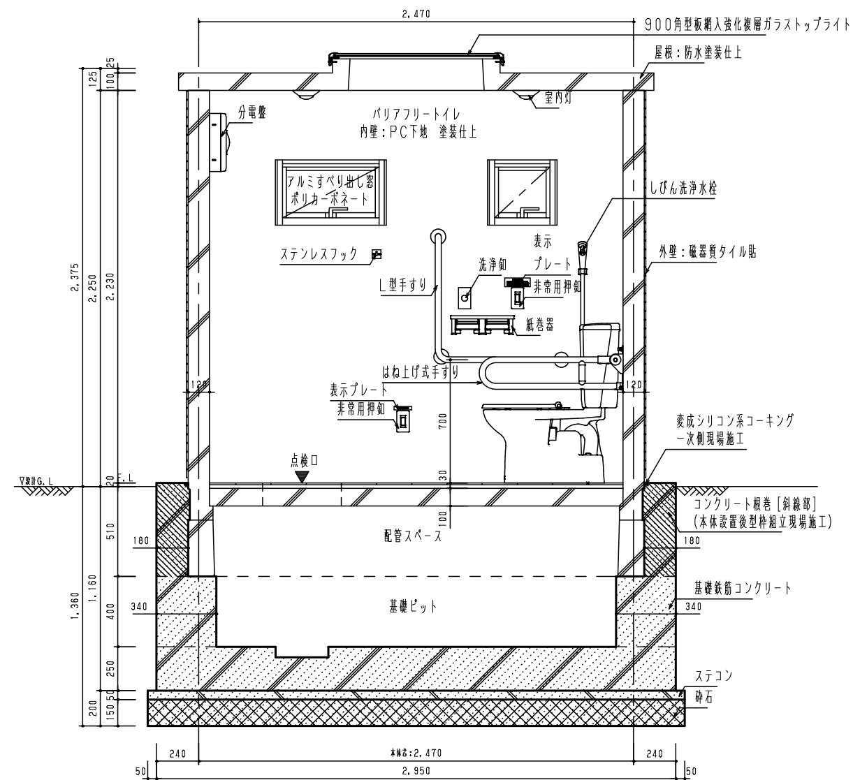
A - A' 断面詳細図 S = 1 / 30
