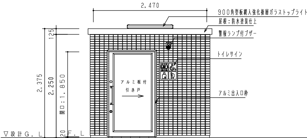
正面図 S = 1 / 5 0
