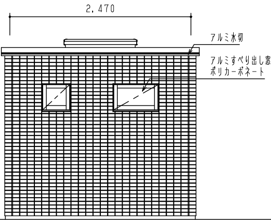
背面図 S = 1 / 5 0
