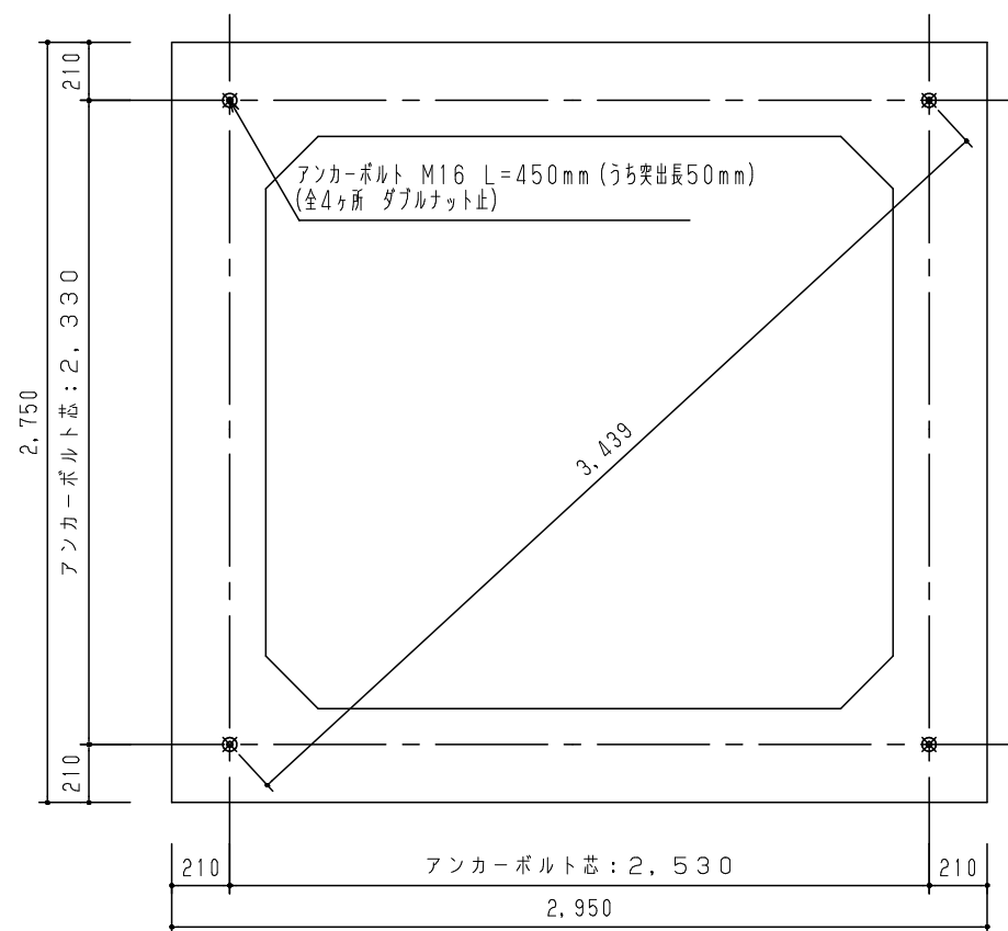
アンカーボルト配置図 S = 1 / 30
