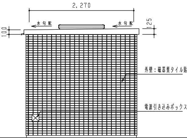
側面図 S = 1 / 5 0
