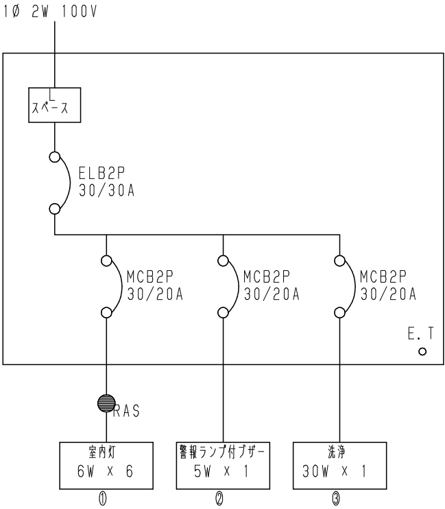
盤 結 線 図
