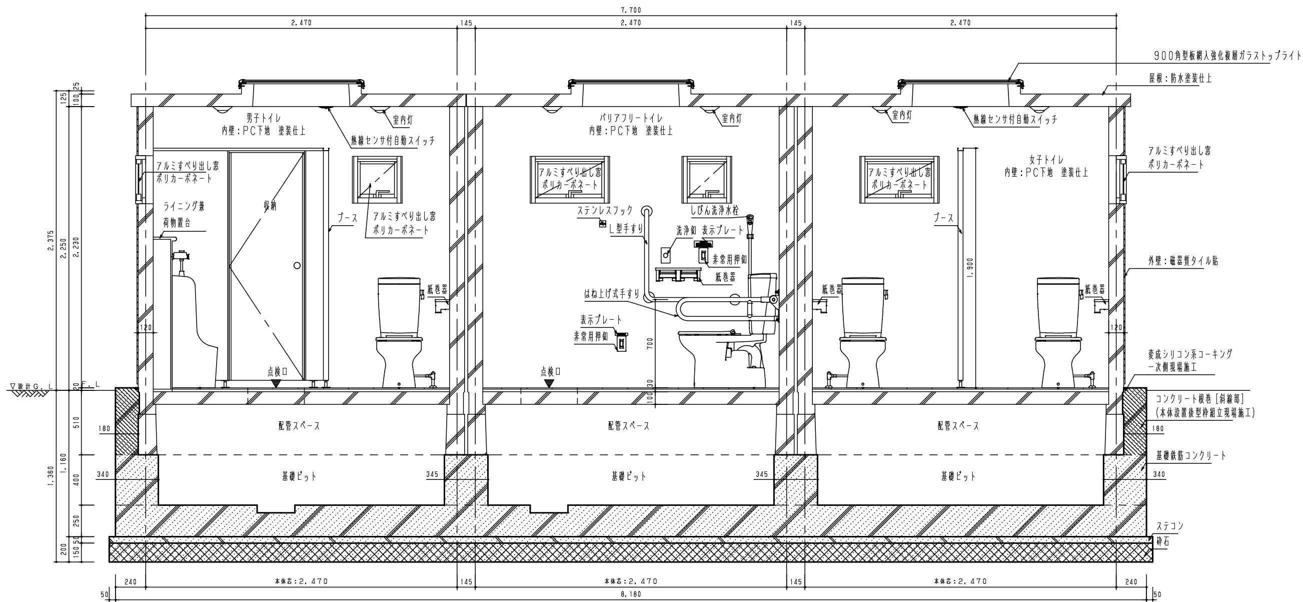
A - A' 断面詳細図 S = 1 / 30 [Hatched Box] 部分は一次側現場施工とする。
