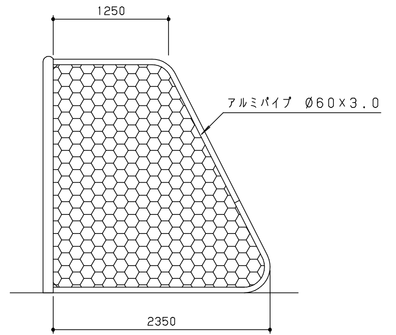
側面図 S = 1 / 40
