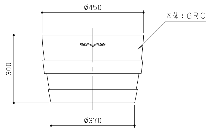
側面図 S = 1 / 10
