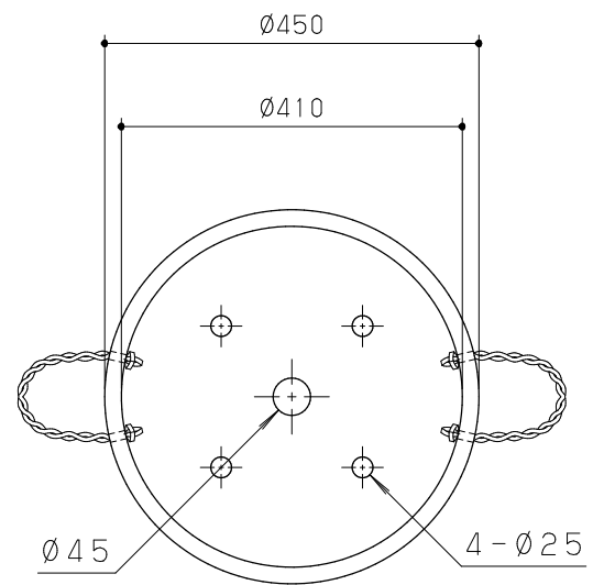
平面図 S = 1 / 10
