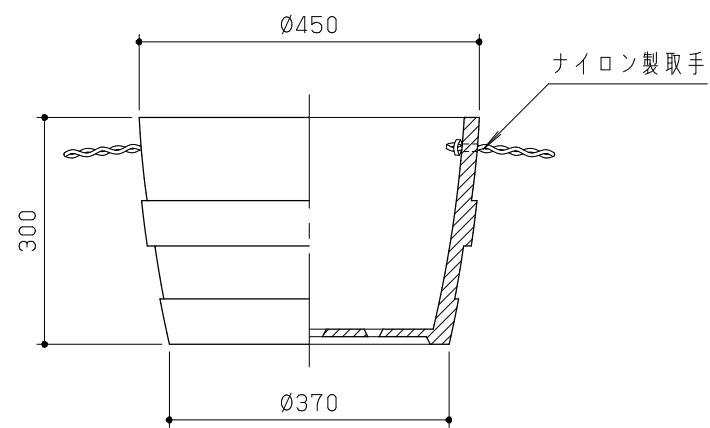
立・断面図 S = 1 / 10
