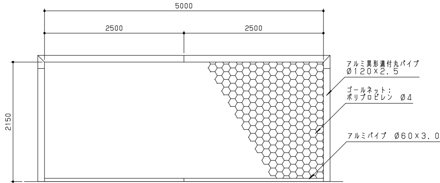
正面図 S = 1 / 40
