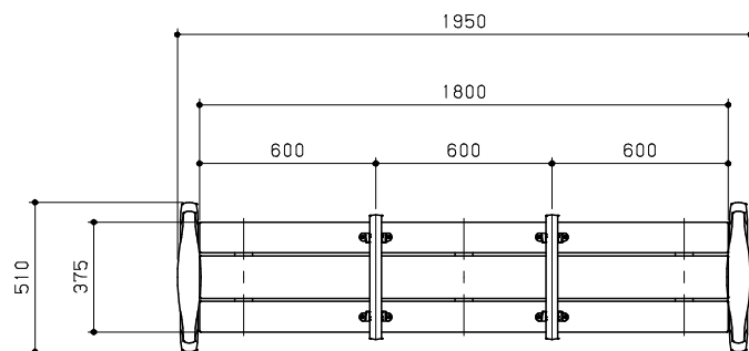
平面図 S = 1 / 20
