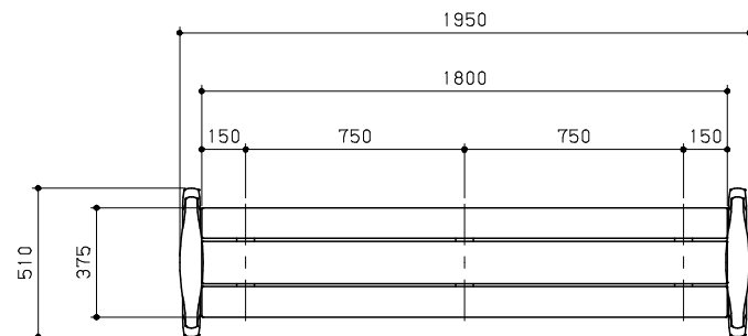
平面図 S = 1 / 20
