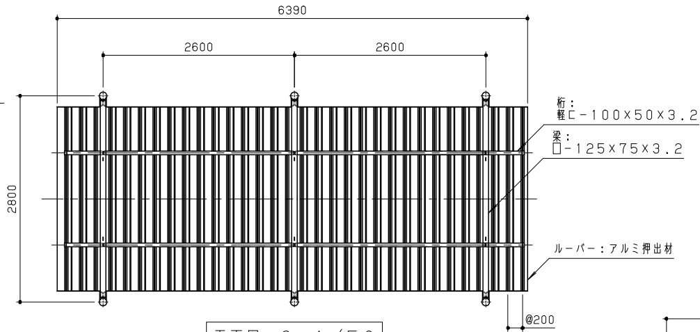
平面図 S = 1/50
