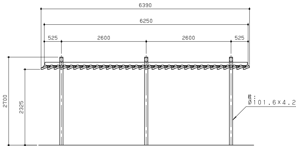
立面図 S = 1/50
