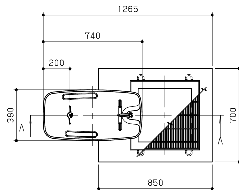
平面図 S=1/20
