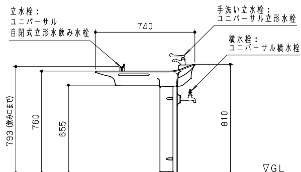
立面図 S=1/20
