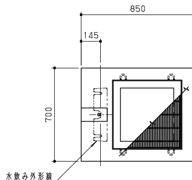
配置図 S=1/20
