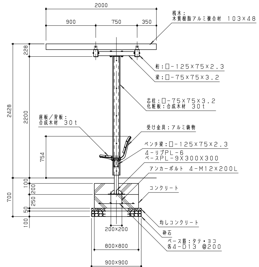
断面図 S = 1 / 30
