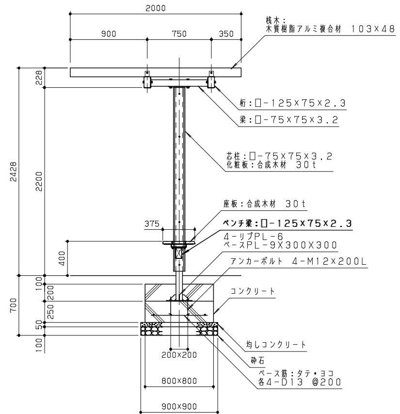
断面図 S = 1 / 30
